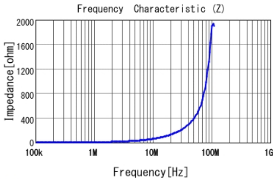
■ LQM2HPN1R0MJ0 |Z|
