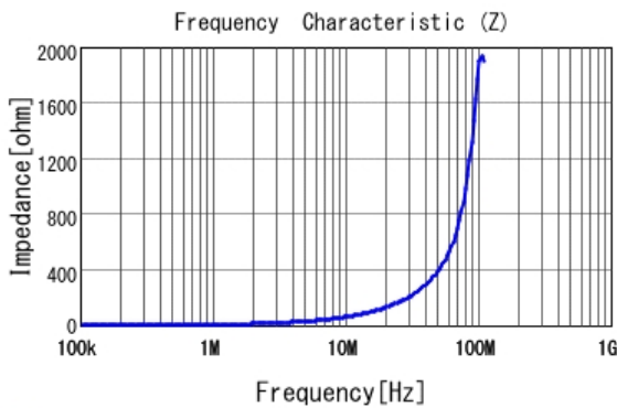
LQM2HPZ1R0MJ0 |Z|
