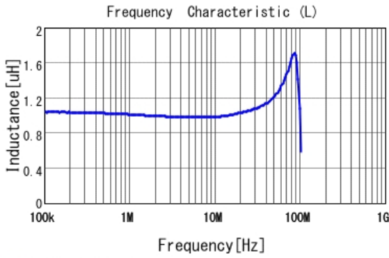
LQM2HPZ1R0MJ0 L
