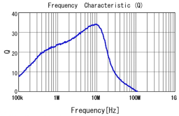
LQM2HPZ1R0MJ0 Q
