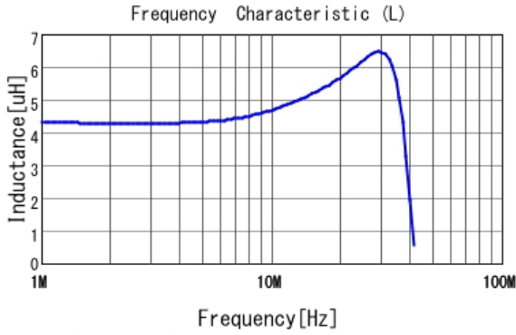
■ LQM2HPZ4R7MGC L
