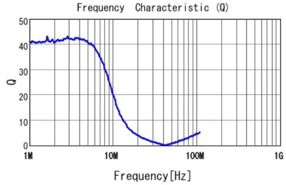
■ LQM2HPZ4R7MGC Q
