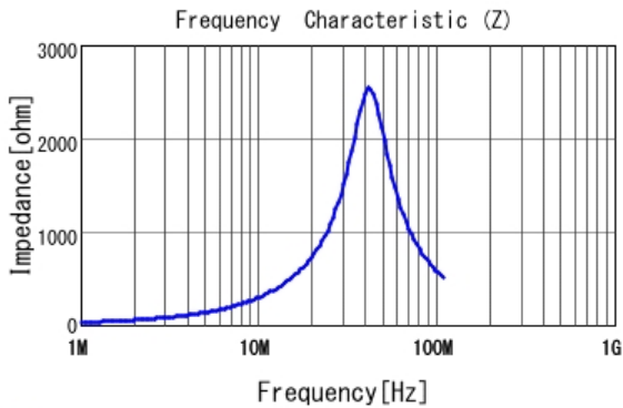
■ LQM2HPZ4R7MGC |Z|
