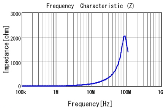
■ LQM2MPN1R5MG0 |Z|
