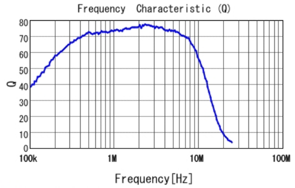
■ LQM2MPN4R7NG0 Q
