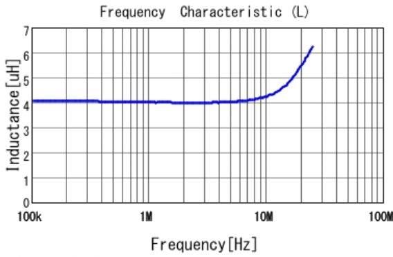
■ LQM2MPN4R7NG0 L
