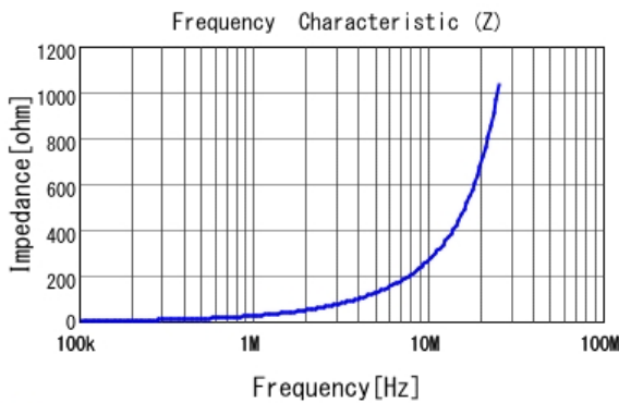
■ LQM2MPN4R7NG0 |Z|
