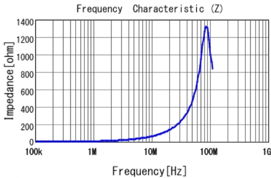
■ LQM31PN1R0M00 |Z|
