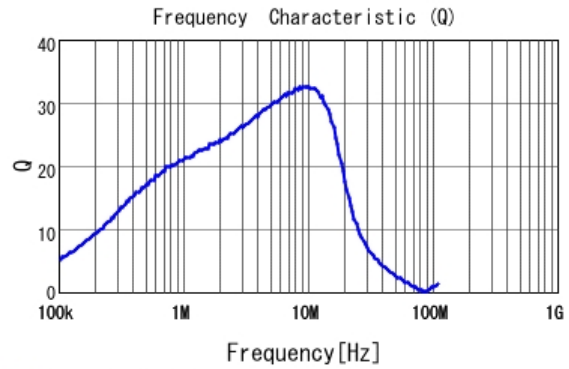
■ LQM31PN1R0M00 Q
