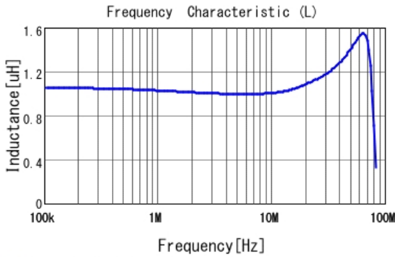
■ LQM31PN1R0M00 L
