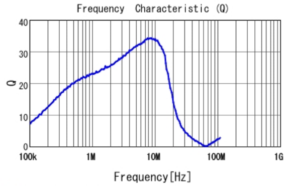
■ LQM31PN2R2M00 Q
