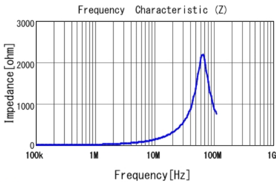
■ LQM31PN2R2M00 |Z|
