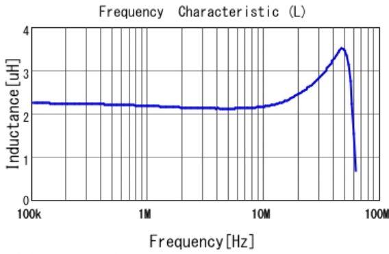
■ LQM31PN2R2M00 L
