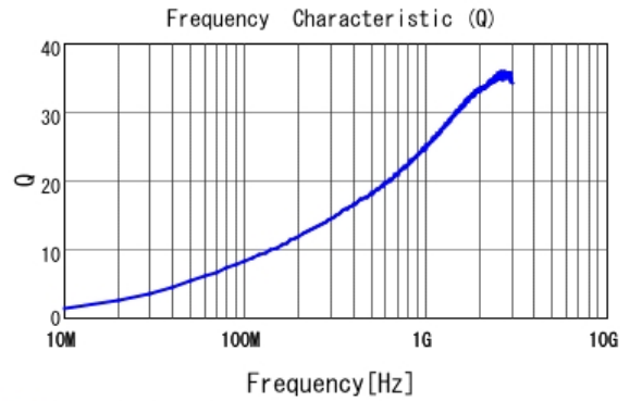
■ LQP02HQ12NJ02 Q
