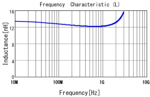
■ LQP02HQ12NJ02 L
