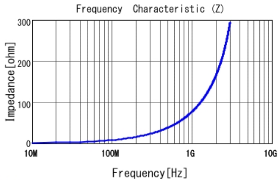
■ LQP02HQ12NJ02 |Z|
