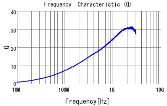
■ LQP02HQ18NH02 Q
