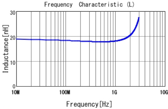
■ LQP02HQ18NH02 L
