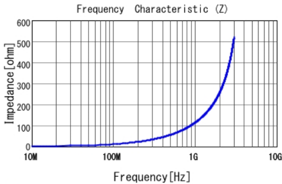
■ LQP02HQ18NH02 |Z|
