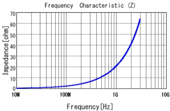
■ LQP02HQ3N3B02 |Z|
