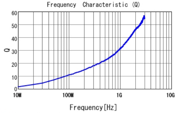
■ LQP02HQ3N3B02 Q
