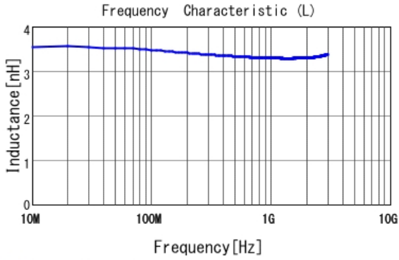
■ LQP02HQ3N3B02 L
