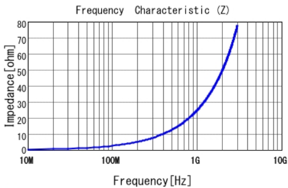
■ LQP02HQ3N9B02 |Z|
