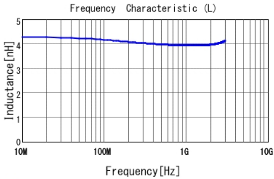
■ LQP02HQ3N9B02 L
