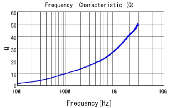
■ LQP02HQ3N9B02 Q
