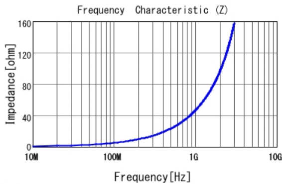
■ LQP02HQ7N5H02 |Z|
