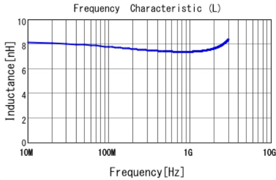
■ LQP02HQ7N5H02 L
