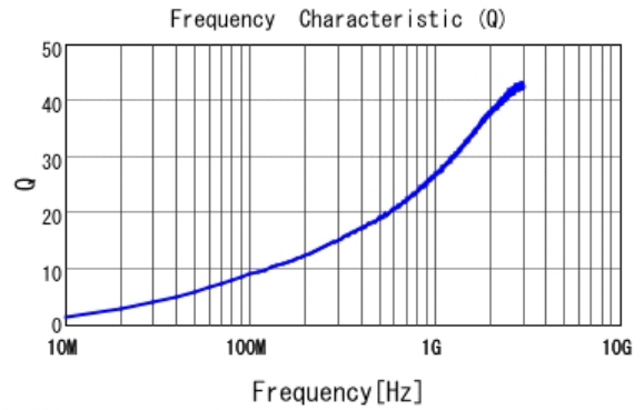
■ LQP02HQ7N5H02 Q
