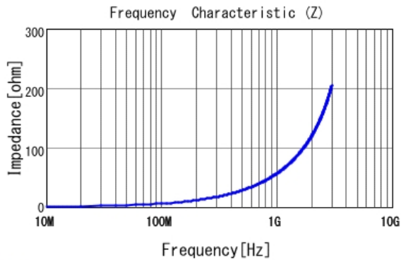
■ LQP02HQ9N1H02 |Z|
