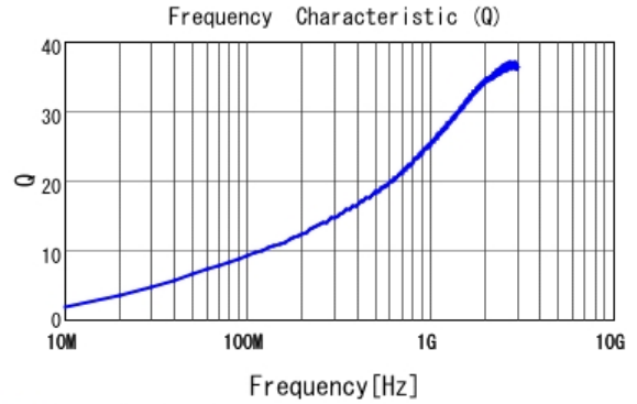
■ LQP02HQ9N1H02 Q
