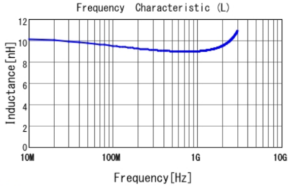
■ LQP02HQ9N1H02 L
