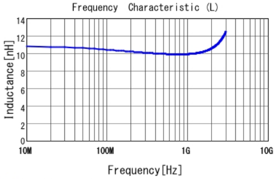
■ LQP02TN10NH02 L
