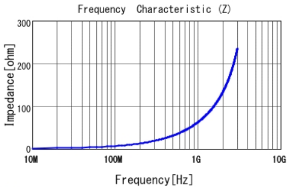
■ LQP02TN10NH02 |Z|
