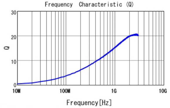
■ LQP02TN10NH02 Q
