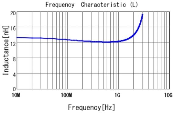
■ LQP02TN12NH02 L
