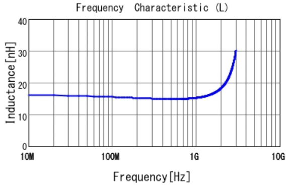
■ LQP02TN15NH02 L
