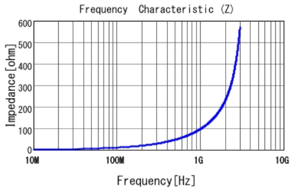
■ LQP02TN15NH02 |Z|
