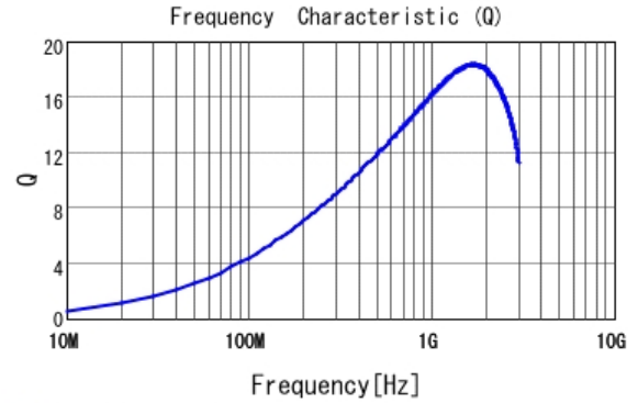
■ LQP02TN15NH02 Q
