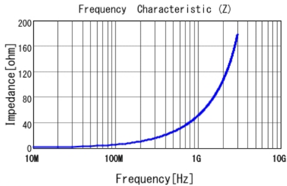
■ LQP02TN8N2H02 |Z|
