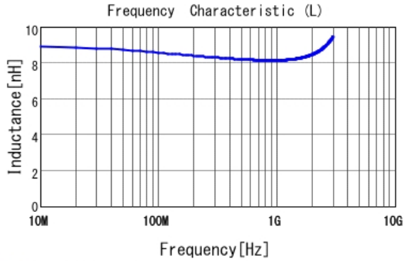
■ LQP02TN8N2H02 L
