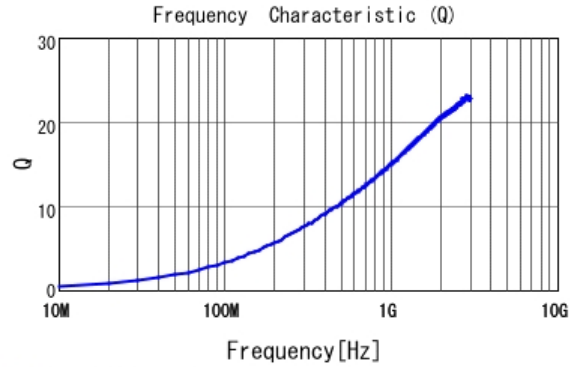
■ LQP02TN8N2H02 Q
