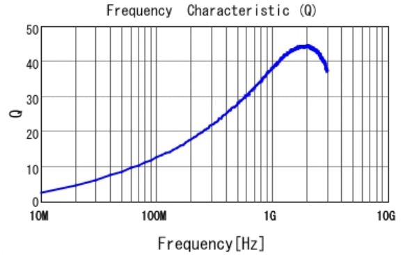
■ LQP03HQ12NJ02 Q
