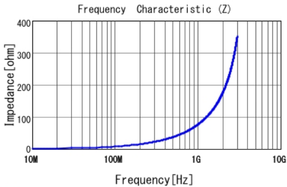
■ LQP03HQ12NJ02 |Z|
