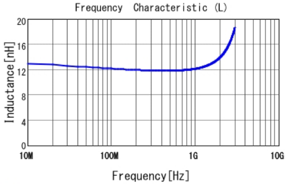
■ LQP03HQ12NJ02 L
