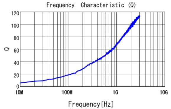
■ LQP03HQ1N2B02 Q
