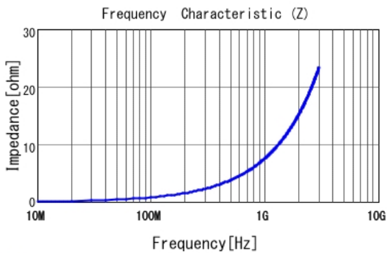
■ LQP03HQ1N2B02 |Z|
