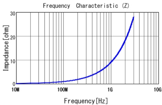
■ LQP03HQ1N4B02 |Z|
