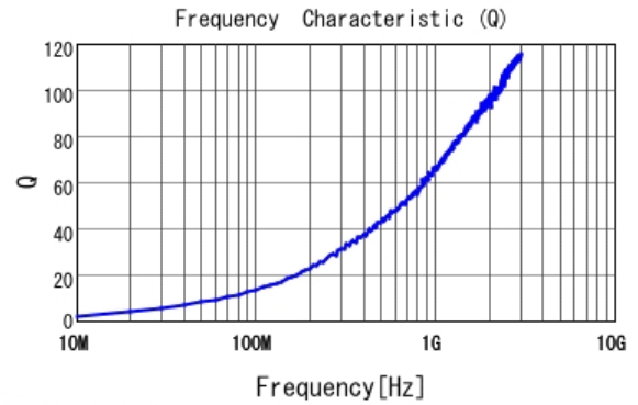
■ LQP03HQ1N4B02 Q
