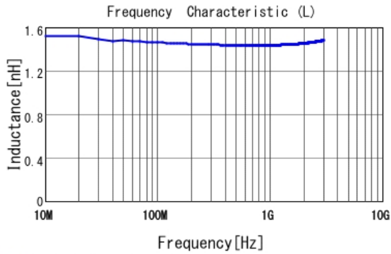
■ LQP03HQ1N4B02 L
