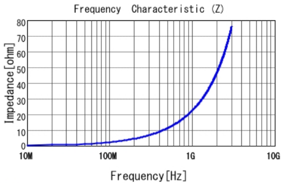
■ LQP03HQ3N6B02 |Z|
