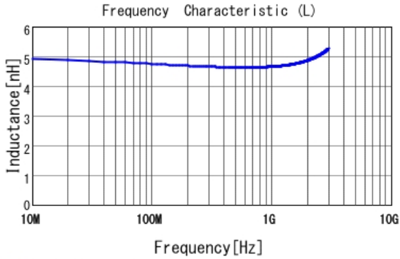
■ LQP03HQ4N7H02 L
