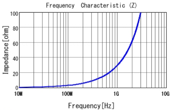
■ LQP03HQ4N7H02 |Z|
