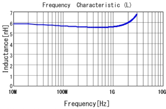
■ LQP03HQ5N6H02 L
