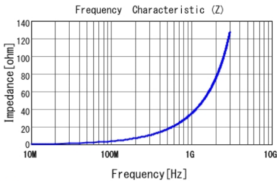
■ LQP03HQ5N6H02 |Z|
