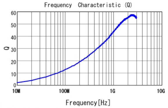
■ LQP03HQ5N6H02 Q
