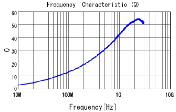
■ LQP03HQ7N5J02 Q
