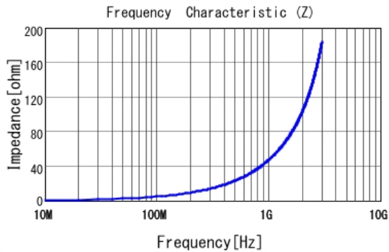
■ LQP03HQ7N5J02 |Z|
