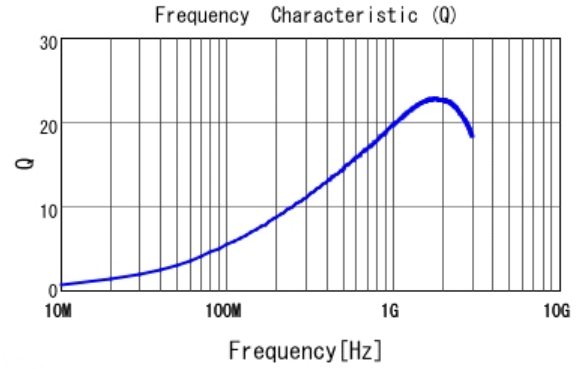
■ LQP03TG10NH02 Q
