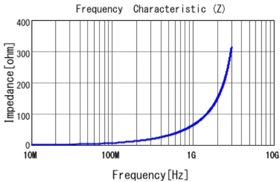
■ LQP03TG10NH02 |Z|
