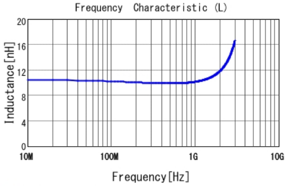
■ LQP03TG10NH02 L
