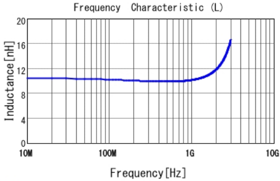
■ LQP03TG10NJ02 L
