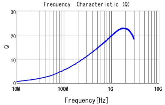
■ LQP03TG10NJ02 Q
