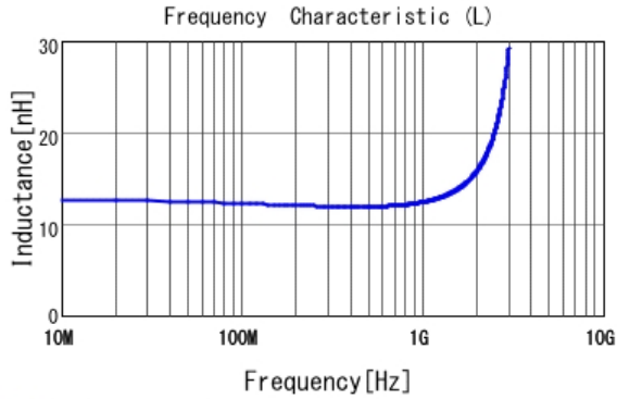
■ LQP03TG12NH02 L
