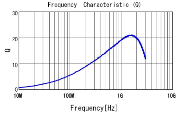
■ LQP03TG12NH02 Q
