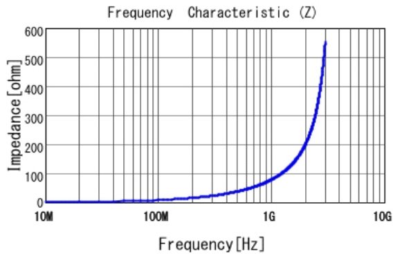
■ LQP03TG12NH02 |Z|
