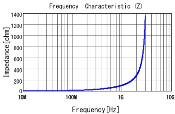
■ LQP03TG15NH02 |Z|
