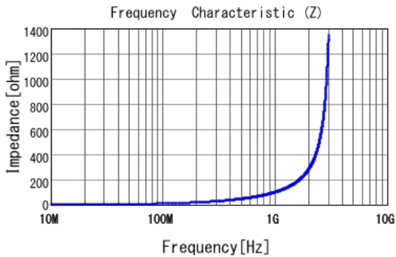
■ LQP03TG15NJ02 |Z|
