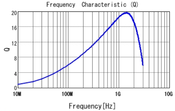
■ LQP03TG15NJ02 Q
