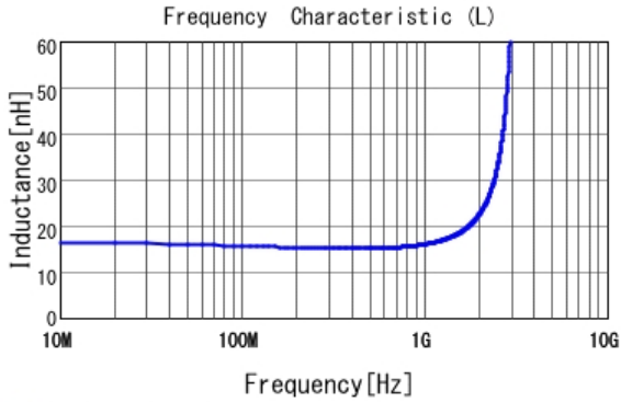
■ LQP03TG15NJ02 L
