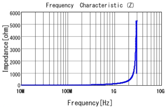
■ LQP03TG18NH02 |Z|
