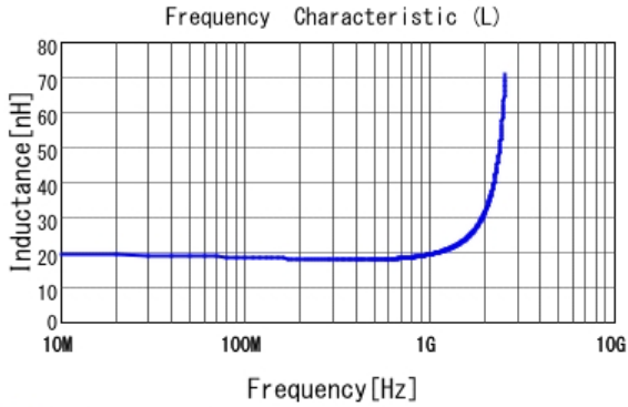
■ LQP03TG18NH02 L
