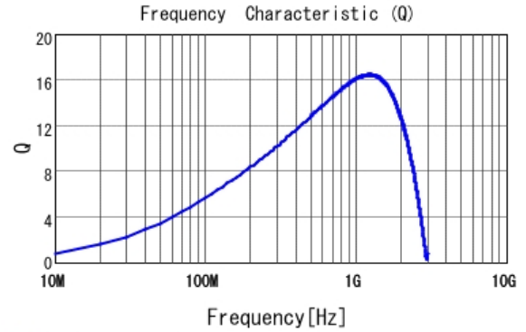
■ LQP03TG18NH02 Q
