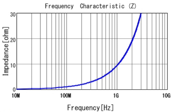
■ LQP03TG1N5B02 |Z|
