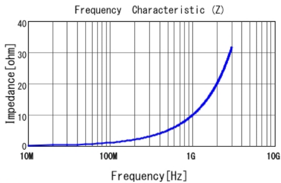
■ LQP03TG1N6B02 |Z|
