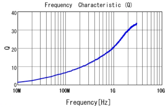
■ LQP03TG1N6B02 Q
