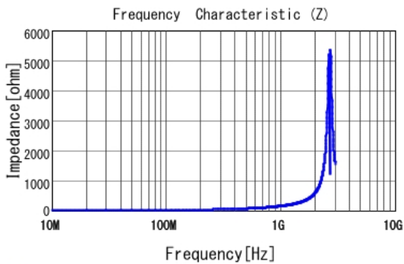
■ LQP03TG22NH02 |Z|
