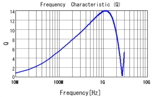
■ LQP03TG22NH02 Q
