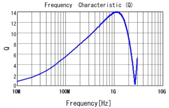
■ LQP03TG22NJ02 Q
