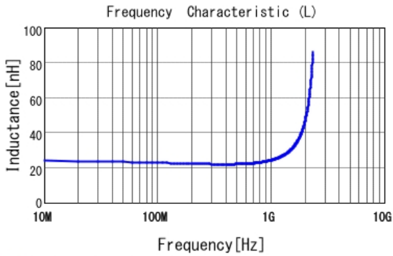
■ LQP03TG22NJ02 L
