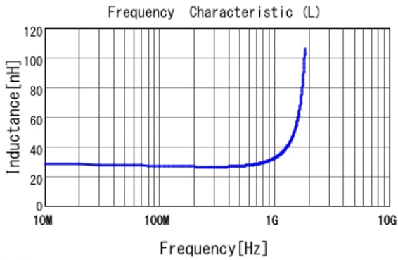
■ LQP03TG27NH02 L
