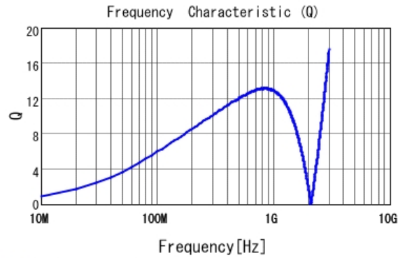
■ LQP03TG27NH02 Q
