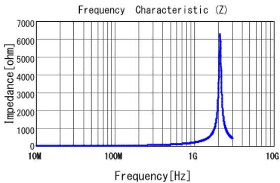
■ LQP03TG27NJ02 |Z|
