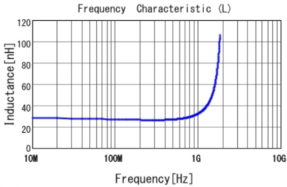
■ LQP03TG27NJ02 L
