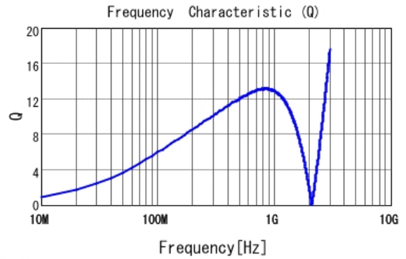
■ LQP03TG27NJ02 Q
