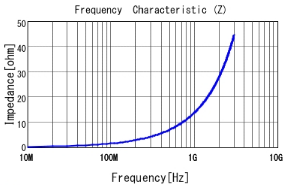
■ LQP03TG2N2B02 |Z|
