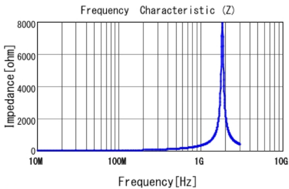
■ LQP03TG39NJ02 |Z|
