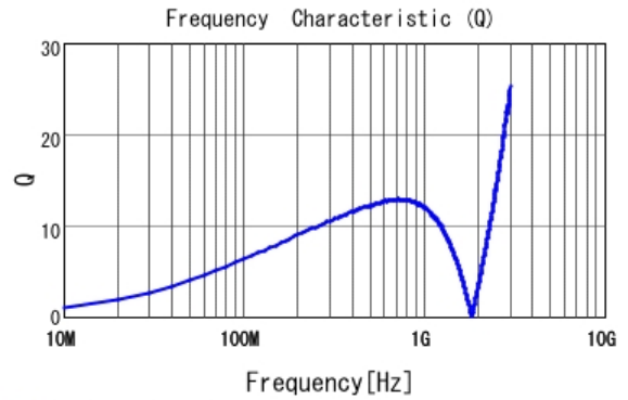
■ LQP03TG39NJ02 Q
