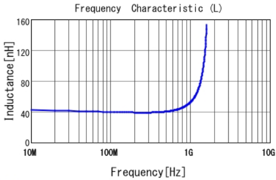
■ LQP03TG39NJ02 L
