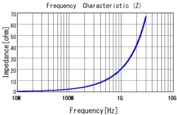
■ LQP03TG3N2B02 |Z|
