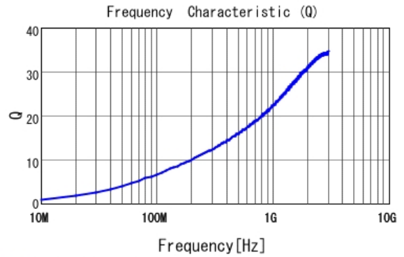
■ LQP03TG3N2B02 Q
