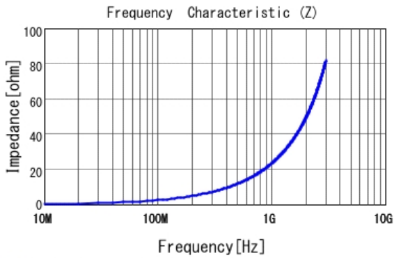
■ LQP03TG3N7B02 |Z|
