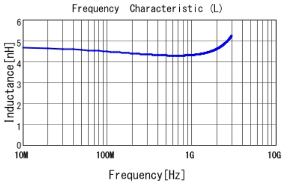
■ LQP03TG4N3H02 L
