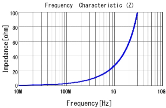
■ LQP03TG4N3H02 |Z|
