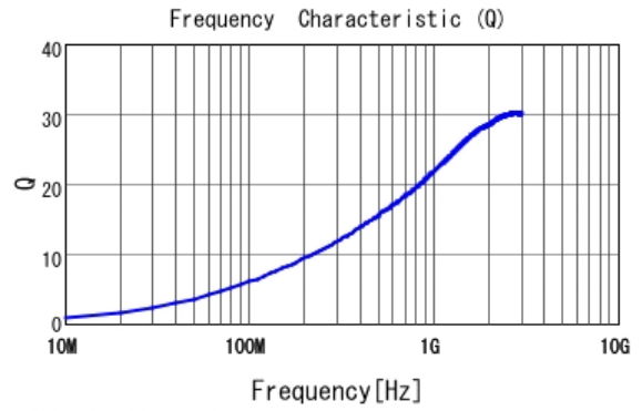
■ LQP03TG4N3H02 Q
