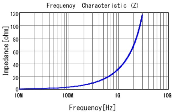
■ LQP03TG5N1H02 |Z|
