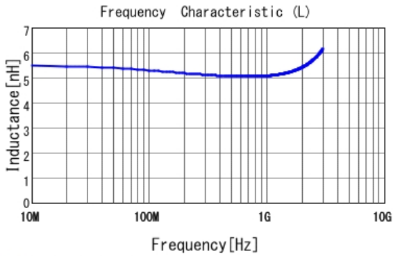
■ LQP03TG5N1H02 L
