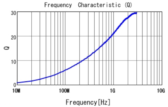
■ LQP03TG5N1H02 Q
