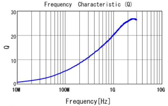
■ LQP03TG5N6H02 Q
