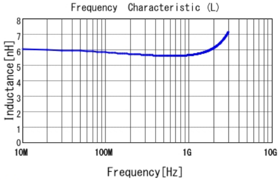
■ LQP03TG5N6H02 L
