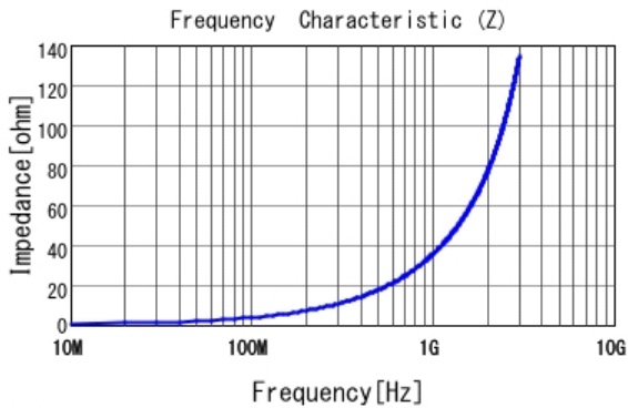
■ LQP03TG5N6H02 |Z|
