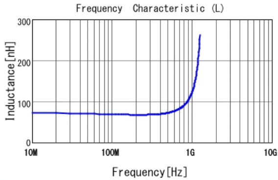
■ LQP03TG68NJ02 L
