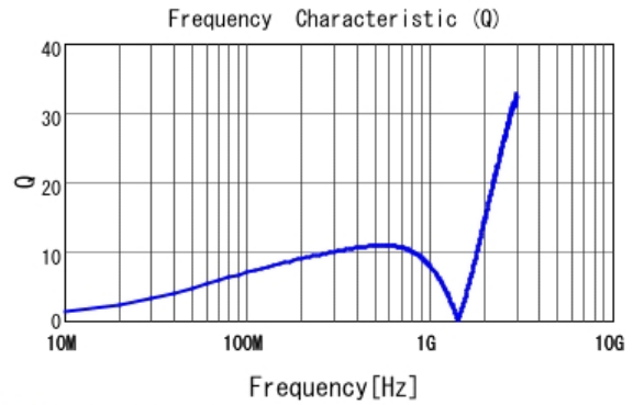
■ LQP03TG68NJ02 Q
