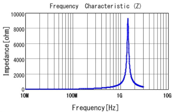
■ LQP03TG68NJ02 |Z|
