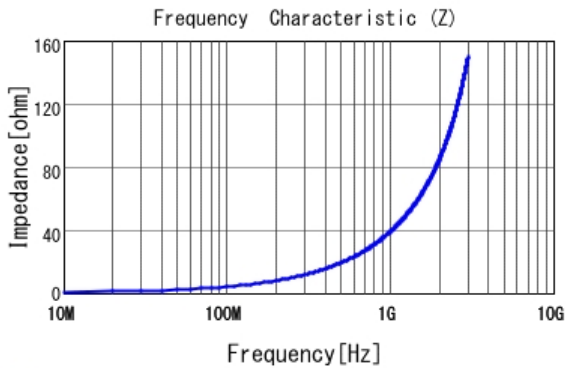
■ LQP03TG6N2H02 |Z|
