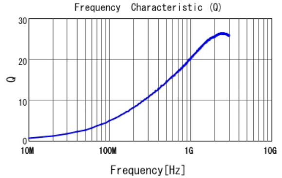
■ LQP03TG6N2H02 Q
