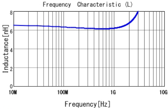
■ LQP03TG6N2H02 L
