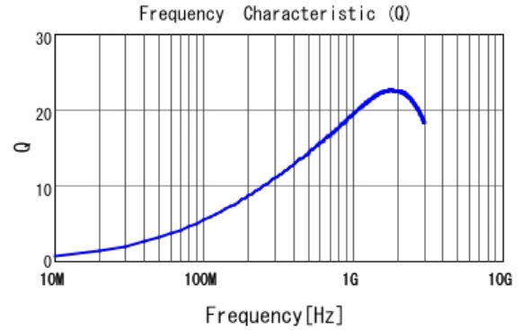
■ LQP03TG9N1H02 Q
