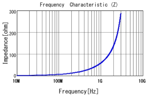
■ LQP03TG9N1H02 |Z|
