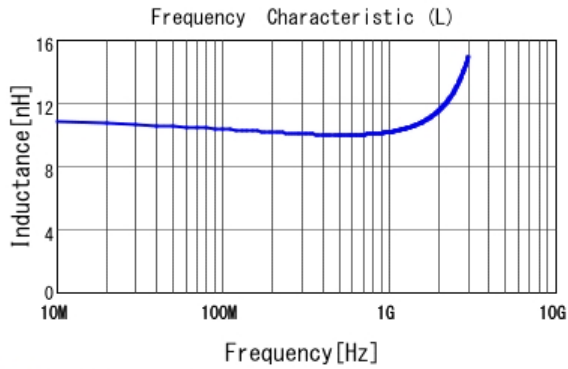
■ LQP03TN10NH02 L
