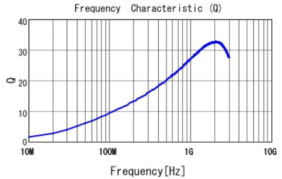
■ LQP03TN10NH02 Q
