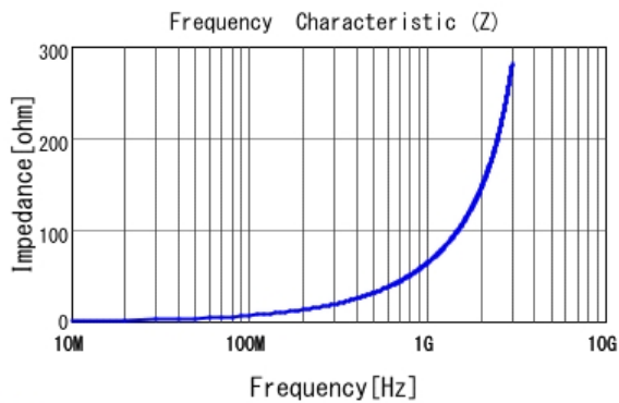
■ LQP03TN10NH02 |Z|
