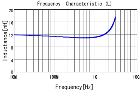
■ LQP03TN11NH02 L
