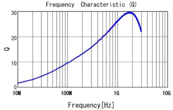
■ LQP03TN11NH02 Q
