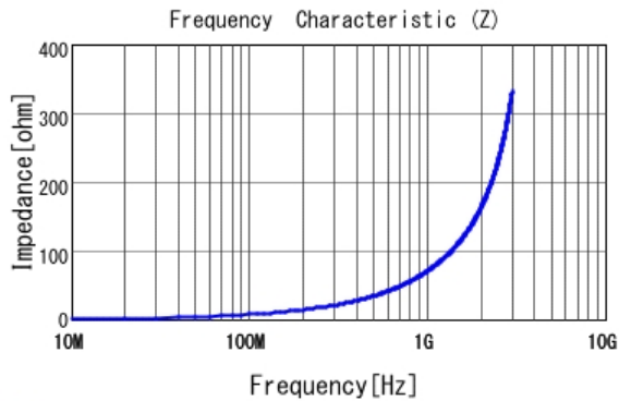
■ LQP03TN11NH02 |Z|
