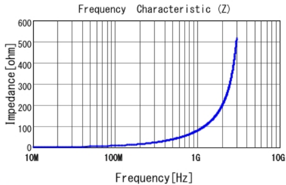
■ LQP03TN12NH02 |Z|
