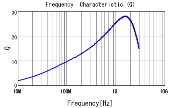
■ LQP03TN12NH02 Q
