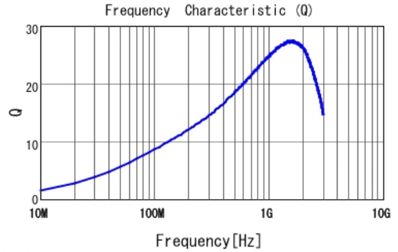
■ LQP03TN13NH02 Q
