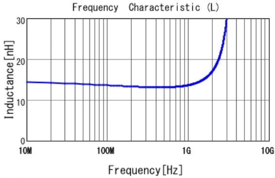
■ LQP03TN13NH02 L
