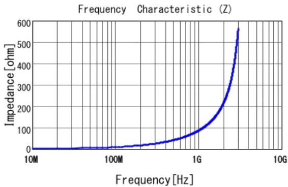
■ LQP03TN13NH02 |Z|
